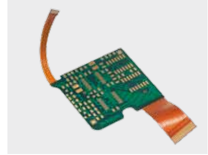
Konturschnitt Starr-Flex-Leiterplatte
