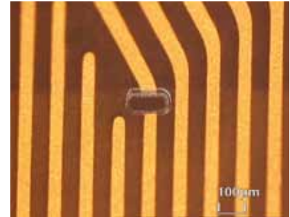
Leiterplattennacharbeit
